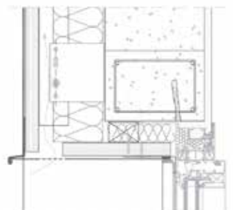
Dintel de ventana ventilada
