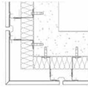
Esquina con panel esquinero
