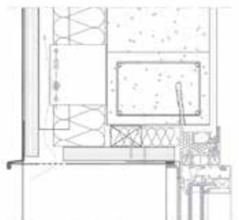
Dintel de ventana ventilada
