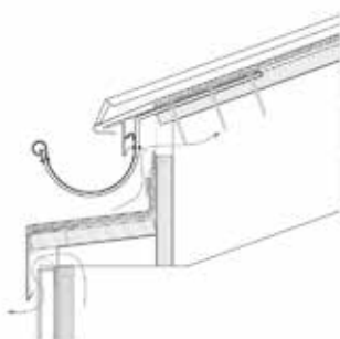
Alero de canalón redondo sobre faldón de zinc
