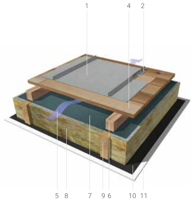
Cubierta ventilada con 'cubierta secundaria'
