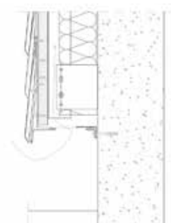
Arranque desde el suelo (teja pico pala)
