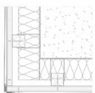
Rincón (teja rombo)
