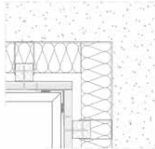
Rincón de esquina - Junta continua
