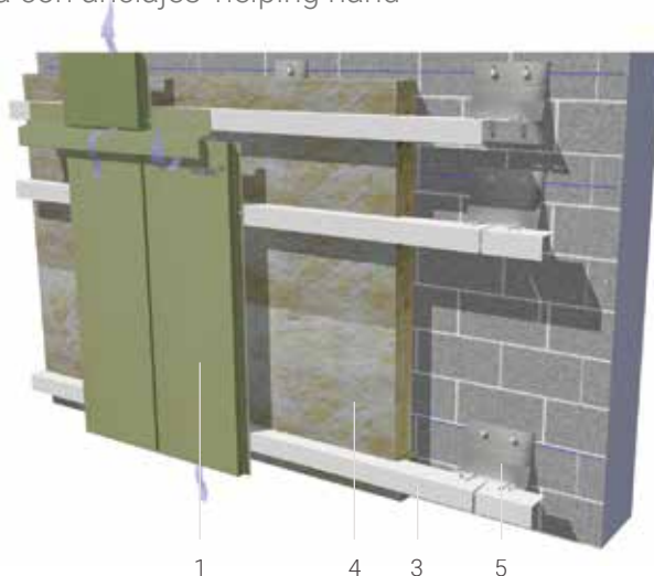
Panel de fachada sobre perfilería metálica horizontal fijada con anclajes 'helping hand'
