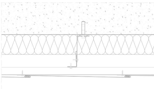
Sección horizontal
