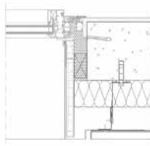
Jamba de ventana
