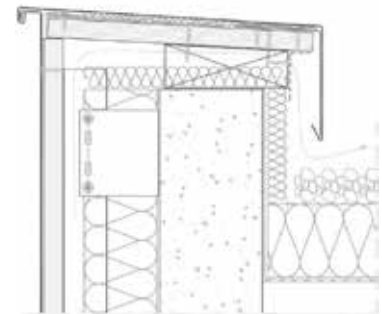
Albardilla ventilada trasera
