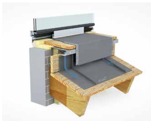
DLSS 6.1.01 – Remate a muro ventilado debajo de ventana.
