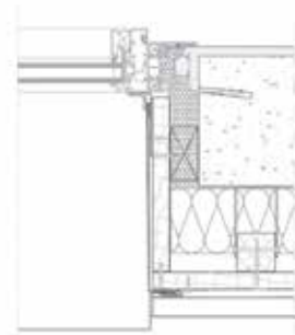
Jamba de ventana
