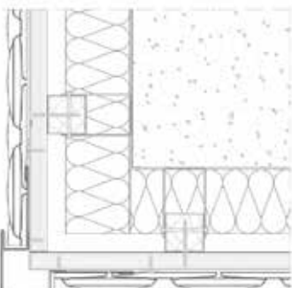
Esquina exterior (teja pico pala)
