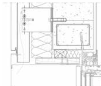
Dintel de ventana ventilada
