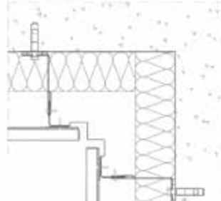
Rincón con perfil rinconero
