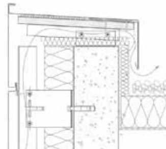
Albardilla ventilada trasera
