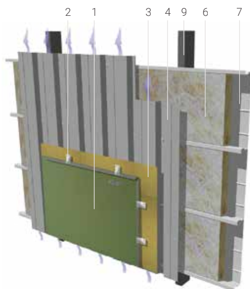
Fachada ventilada sobre bandeja estructural sobre estructura de acero
