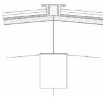
Cumbrera no ventilada de listón cuadrada
