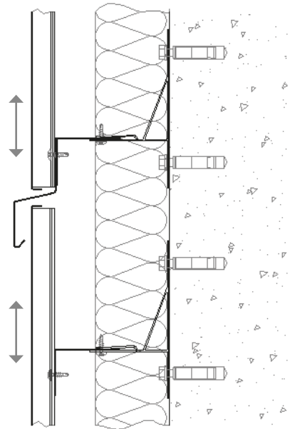
Sección vertical
