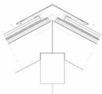
Cumbrera ventilada plana
