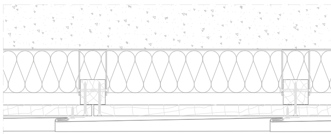
Sección horizontal
