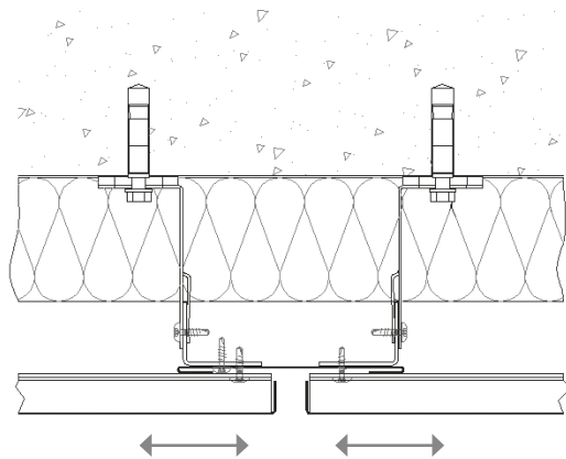
Sección horizontal
