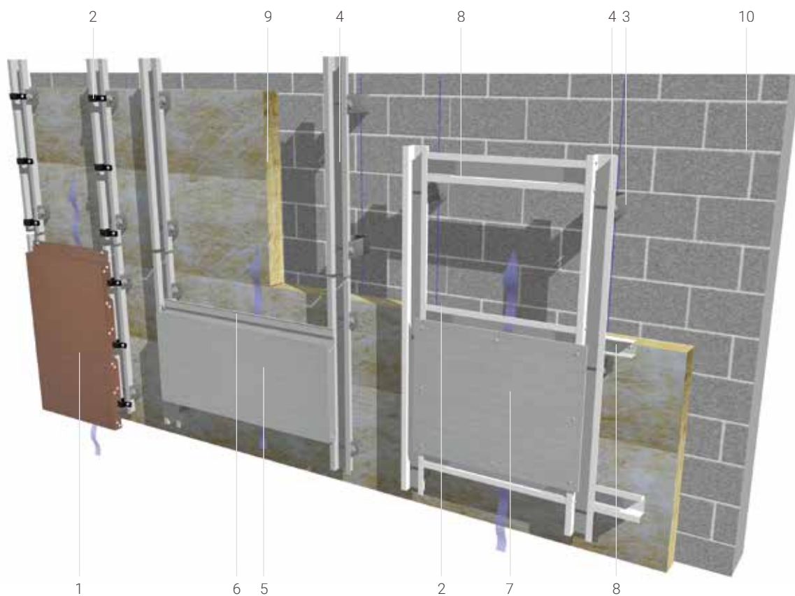
Sistema de casetes colgados, de perfiles machihembrados y de paneles remachados
