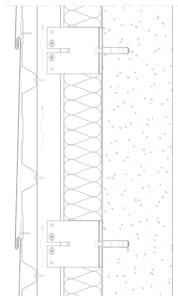
Sección vertical
