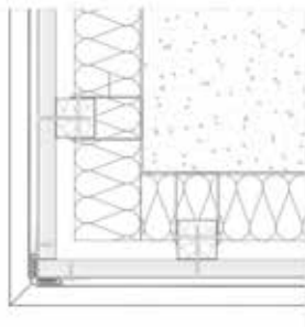
Esquina vertical oculta
