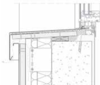
Alfeizar de ventana ventilada
