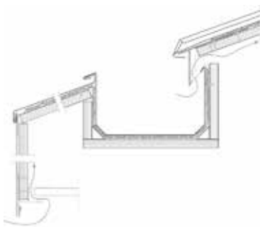
Pesebrón de alero con frontis de zinc
