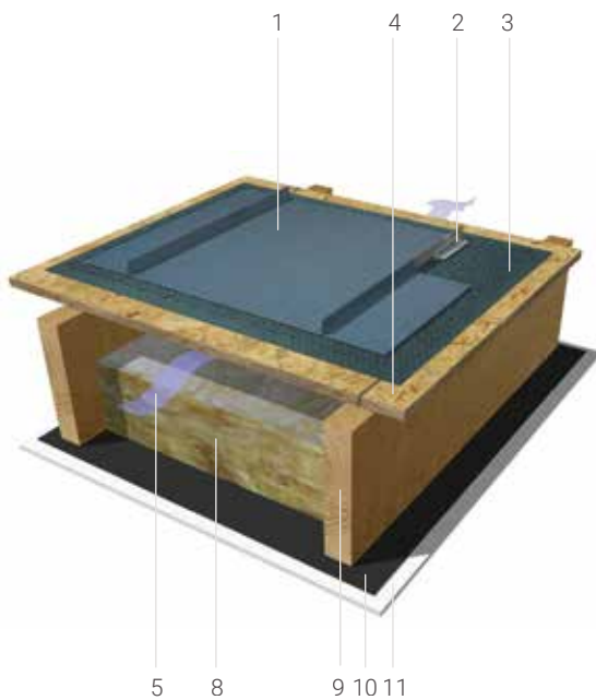
Cubierta ventilada
