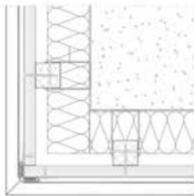
Esquina vertical - Junta continua
