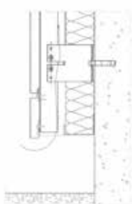
Arranque desde el suelo
