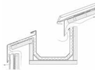
Pesebrón sobre revestimiento de junta alzada en ángulo
