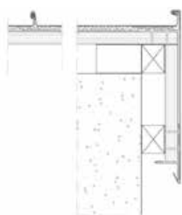
Hastial de junta alzada - Frontis profundo
