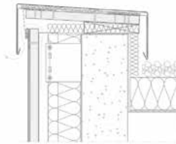
Albardilla ventilada delantera
